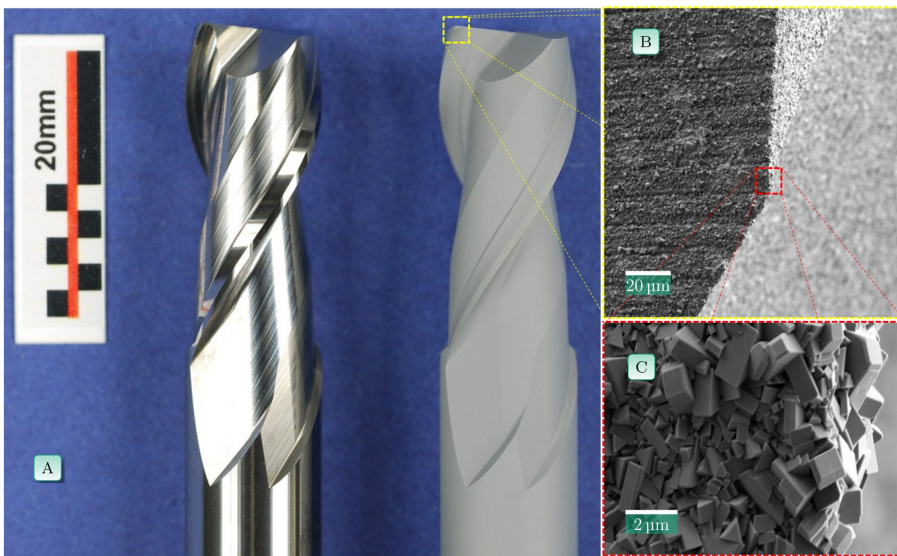
(A) Unbehandelter Fräser (links), behandelter Fräser (rechts); (B/C) Detailaufnahmen der Werkzeugoberfläche nach der Vorbehandlung; © Fraunhofer IWM.
