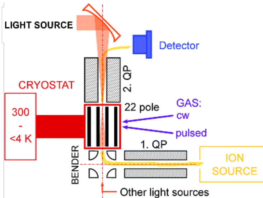
Schematische Darstellung des Versuchsaufbaus zur leak-out spectroscopy
